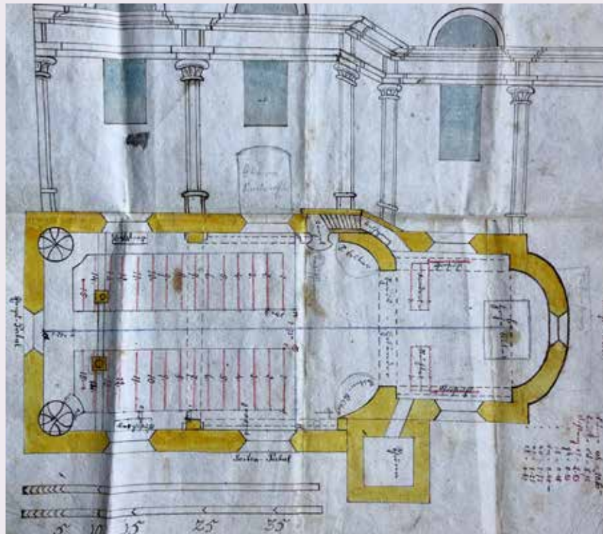
Plan zum Neubau der Kirche
